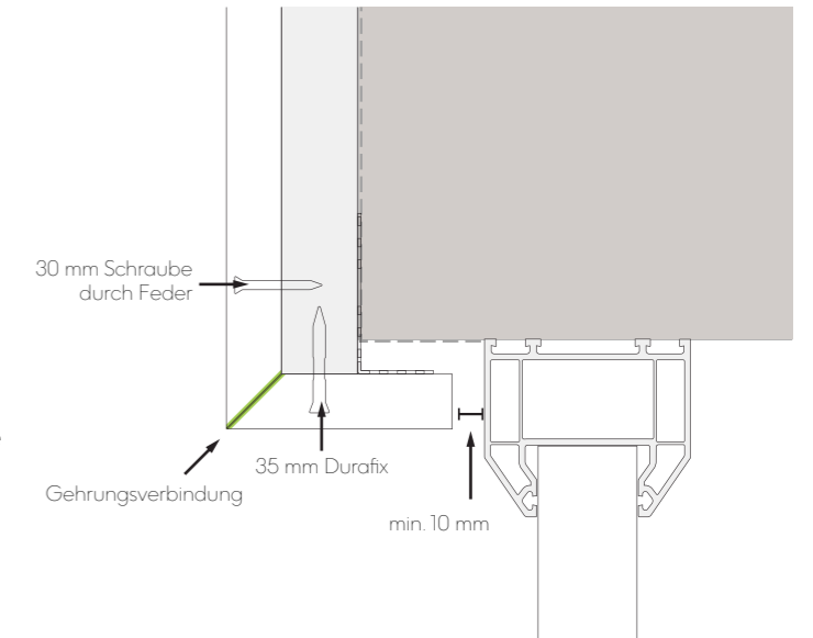
Abb. 14 - Fenster-/Türsturz mit Gehrungsverbindung
