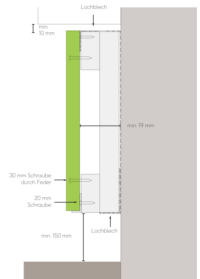
Abb. 1 - Details der oberen und unteren Verkleidung
