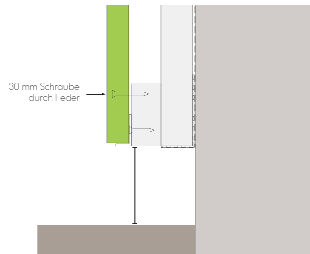
Abb. 17 - Erste Paneelmontage
