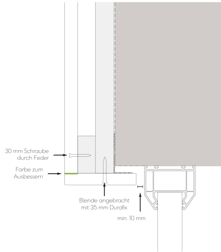
Abb. 12 - Fenster-/Türsturz mit Blende
