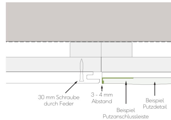
Abb. 19 - Eckprofil stößt an den Putz an
