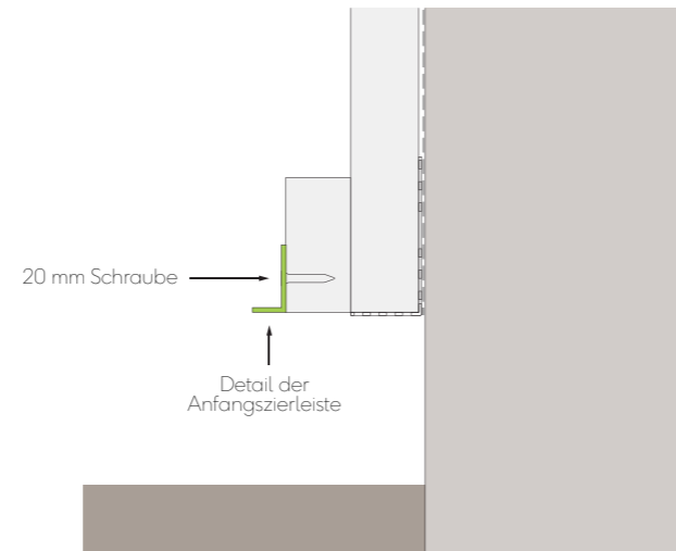
Abb. 16b - Detail der Anfangszierleiste
