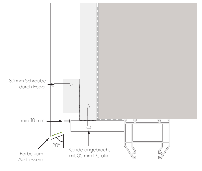
Abb. 15 - Fenster-/Türsturz mit Schrägschnitt
