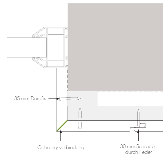
Abb. 13 - Fenster-/Türpfosten mit Gehrungsverbindung
