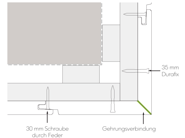
Abb. 10 - Details der auf Gehrung geschnittenen Außenecke
