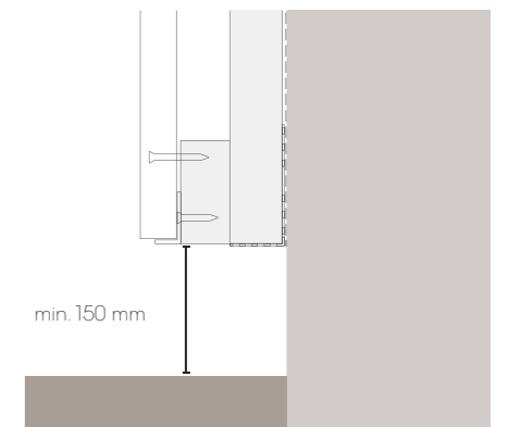
Abb. 4 - Einbaudetail über Bodenhöhe
