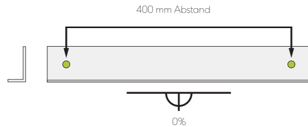
Abb. 16a - Anfangszierleiste
