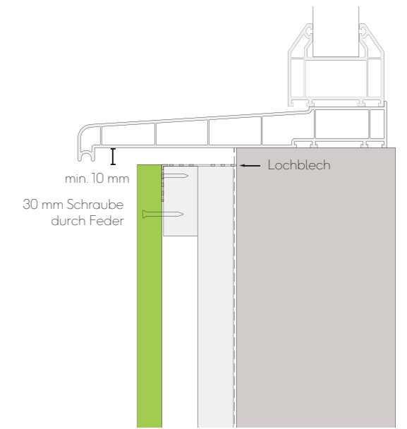
Abb. 3 - Detail Fenster/Türschwelle
