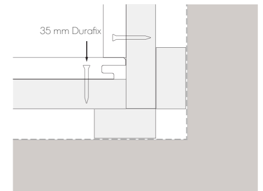
Abb. 9 - Details der Innenstoßecke
