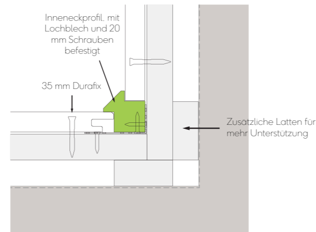
Abb. 7 - Details der Innenecke
