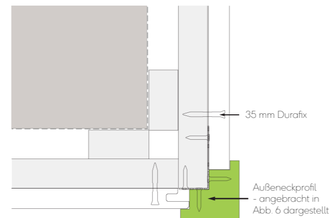
Abb. 8 - Details der Außenecke
